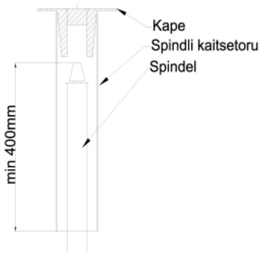
2.18 Veearvesti kaevu põhimõtteskeem ja mõõdud on toodud Lisas I
